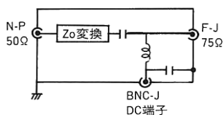
回路図 Circuit PD264
