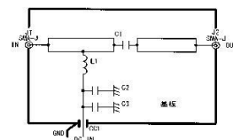
回路図 Circuit PD456
